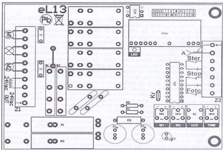
Rys. nr 8. Rozmieszczenie regulatorów na płytce sterownika eL-13.
